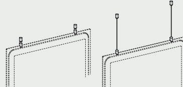
300.KT.05.00 Variante per fissaggio a soffitto /Ceiling fixing variant
